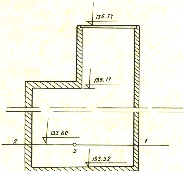
Чертеж колодца М 1:25
