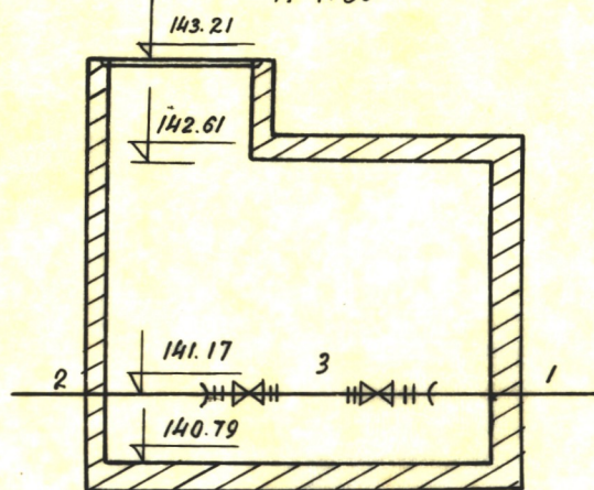
Чертеж колодца М 1:50
