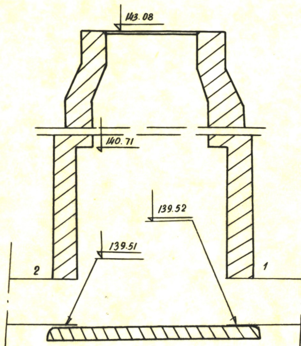
Чертеж колодца М 1:25
