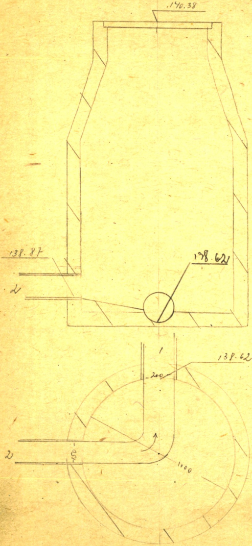
Чертеж колодца М 1:
