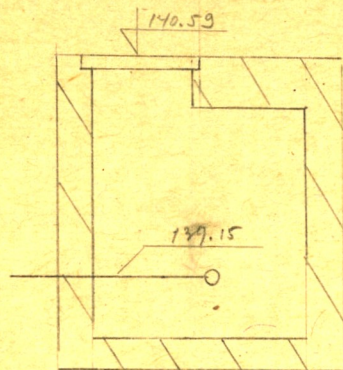
Чертеж колодца М 1:
