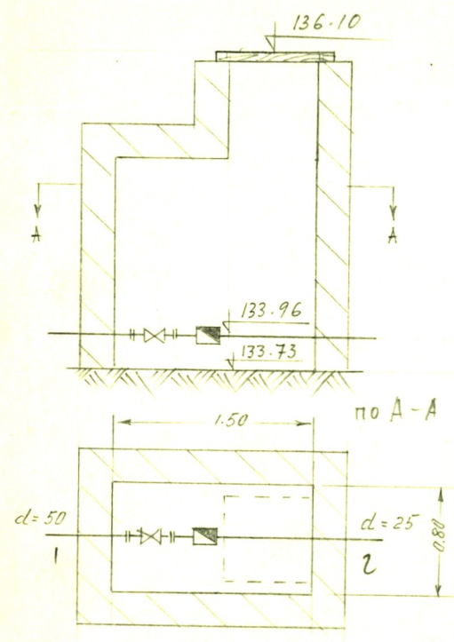
Чертеж колодца М. 1:50
