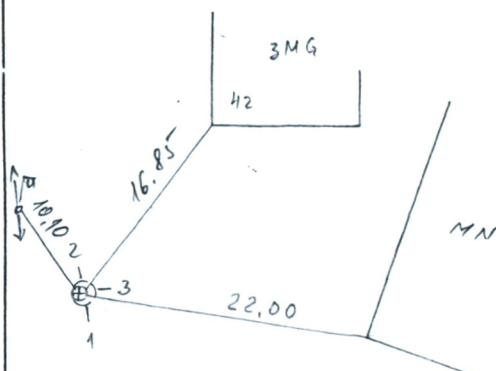
PRIRIŠIMO SCHEMA
