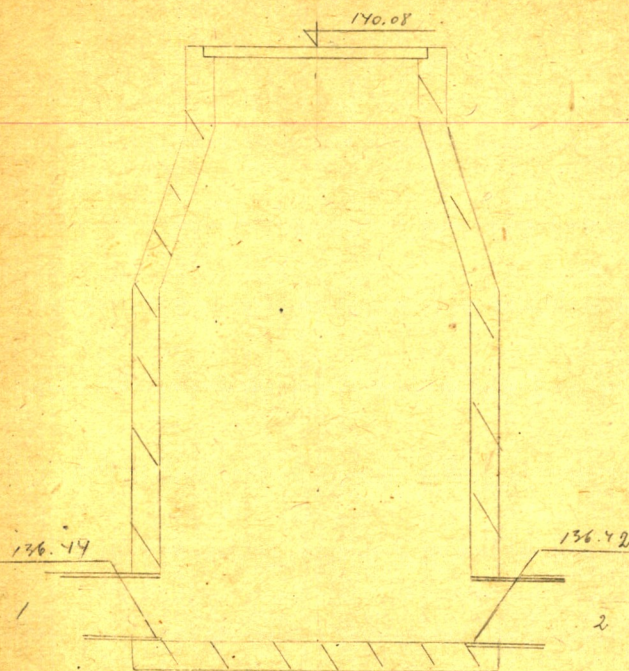
Чертеж колодца М 1:25
