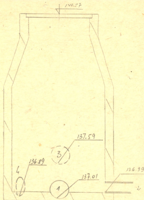
Чертеж колодца М 1:
