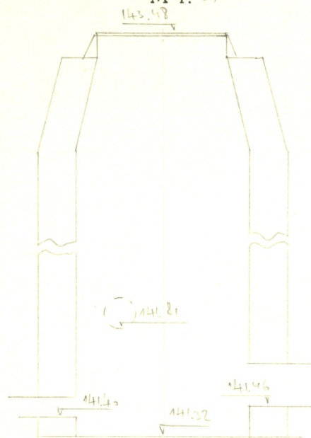
Šulinio brėžinys
