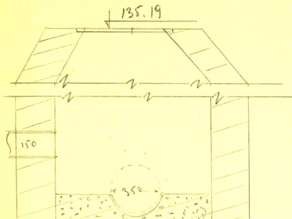
Чертеж колодца М 1:25 по А-А
