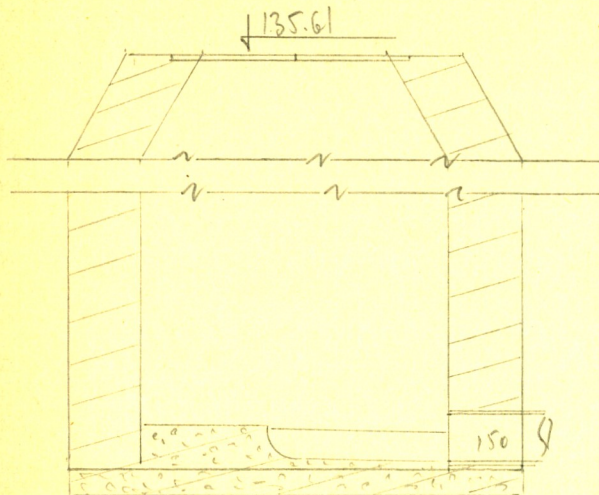
Чертеж колодца М 1:25 по А-А
