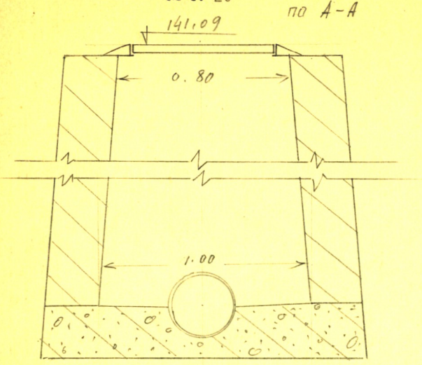
Чертеж колодца М 1: 25
