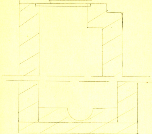
Чертеж колодца по А-А М 1:25 118.71
