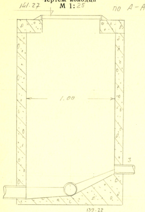
Чертеж колодца М 1:25
