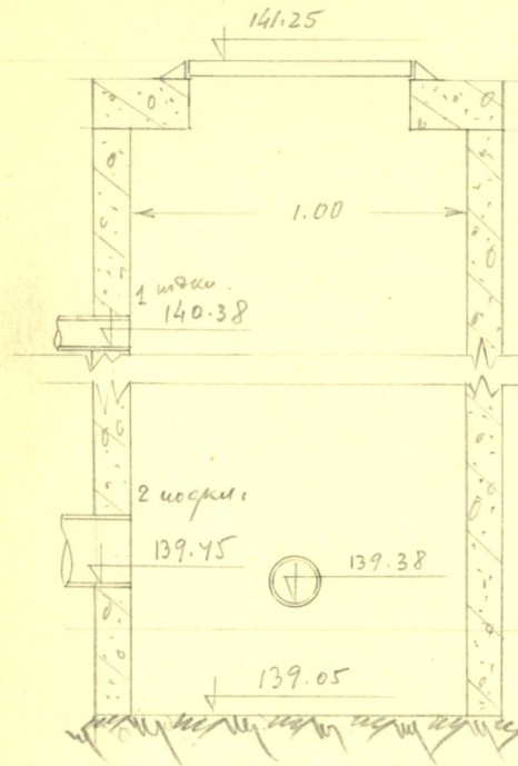
Чертеж колодца М 1:25 по А-А
