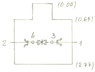
ŠULINIO PIŪVIAI (Matmenys duoti m)
