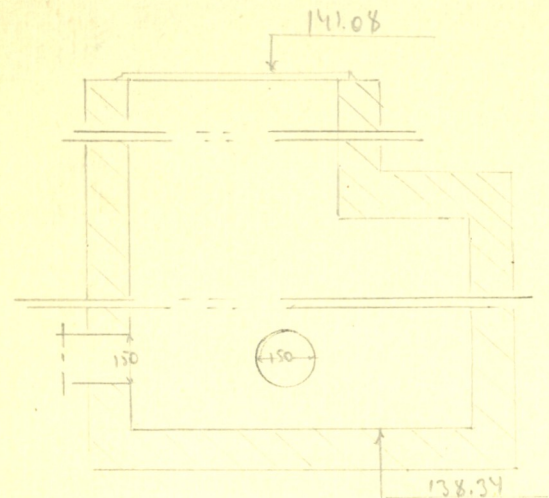
Чертеж колодца М 1:
