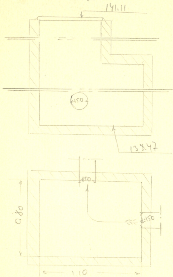
Чертеж колодца М 1:25
