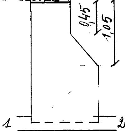
ŠULINIO PIŪVIAI (Matmenys dydžiu m)
