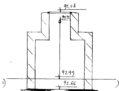
Чертеж колодца М. 1:50
