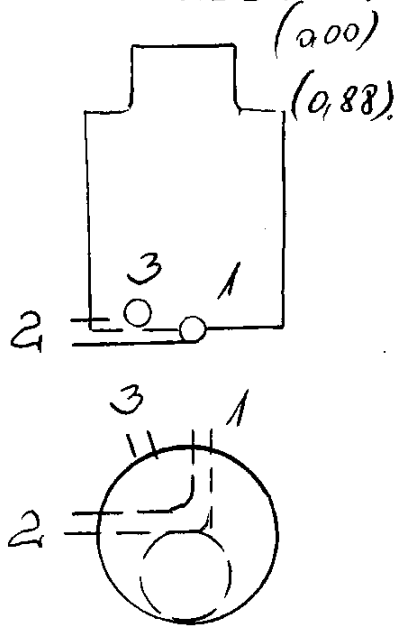
ŠULINIO PIŪVIAI (Matmenys duoti m)
