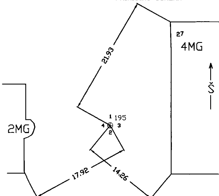
PRIRIŠIMO SCHEMA
