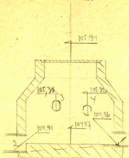
Чертеж колодца М 1: 25
