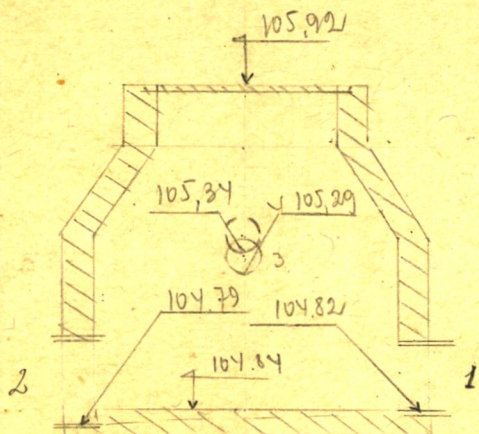
Чертеж колодца М 1:25
