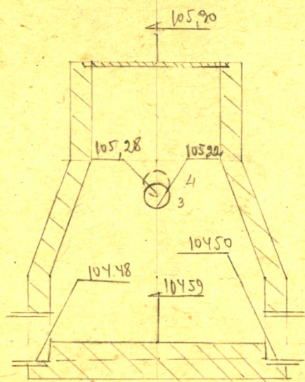
Чертеж колодца М 1: 25
