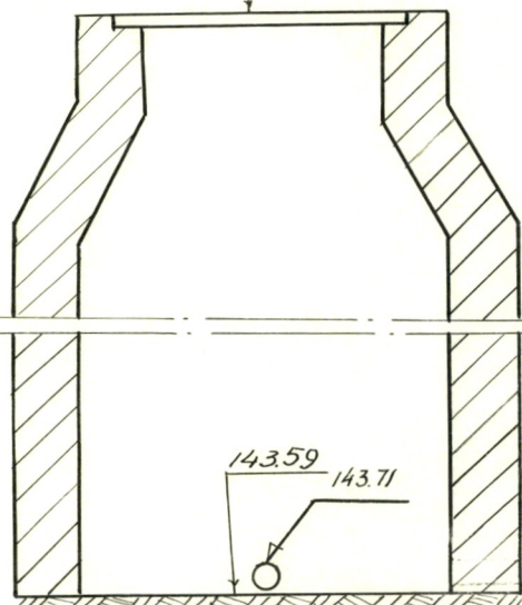
Чертеж колодца М 1:25 145.73
