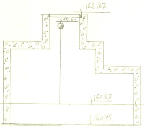
Чертеж колодца М. 1:50
