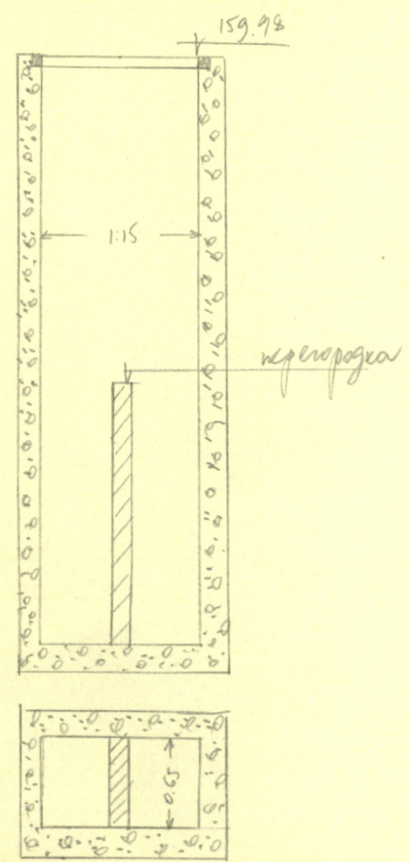
Чертеж колодца М 1:50
