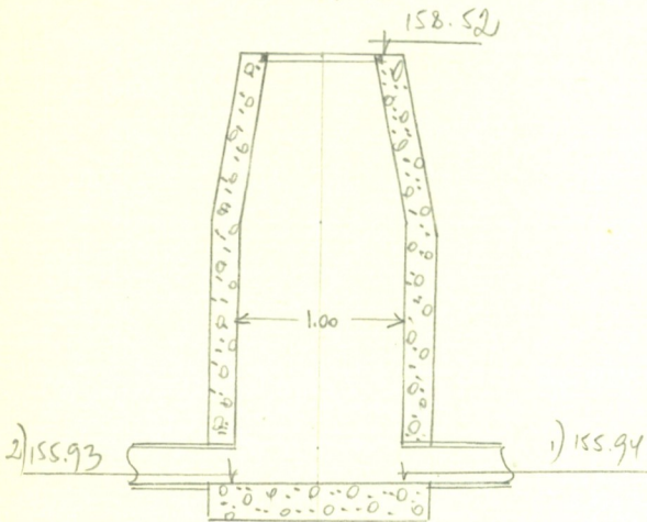
Чертеж колодца М 1:50
