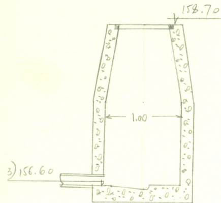
Чертеж колодца М 1:50
