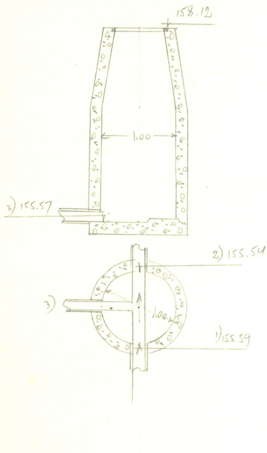
Чертеж колодца М 1:50
