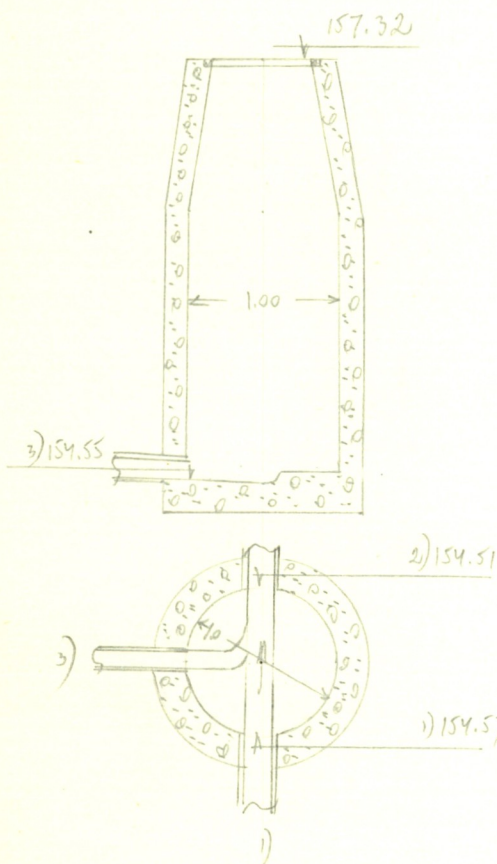
Чертеж колодца М 1:50
