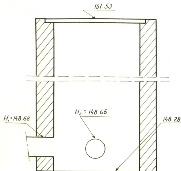
Чертеж колодца М 1:25
