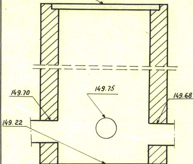
Чертеж колодца М 1:25
