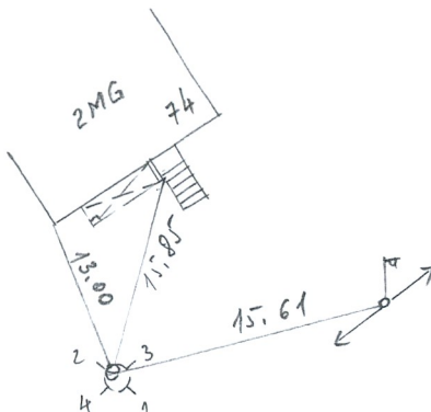
PRIRĖSIMO SCHEMA
