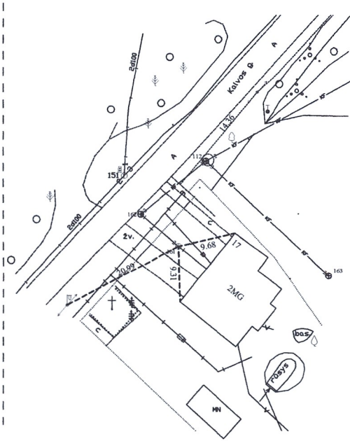
Pririšimo brėžinys
