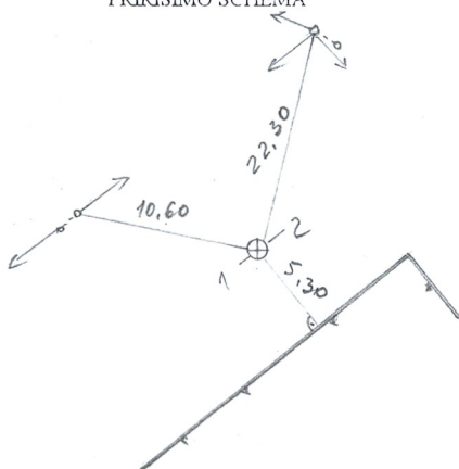
PRIRIŠIMO SCHEMA
