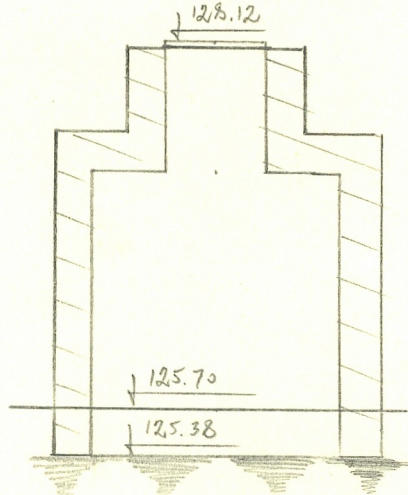
Чертеж колодца М. 1: 50
