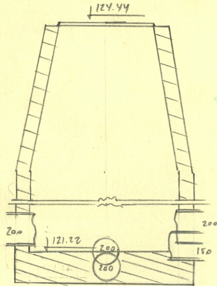
Чертеж колодца М 1:50
