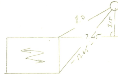
Šulinio kroki
