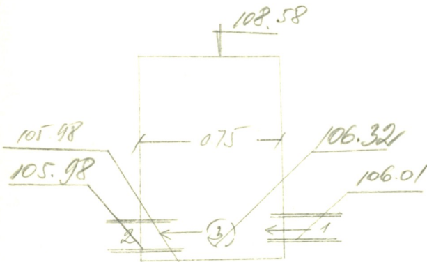
Šulinio brėžinys M 1:
