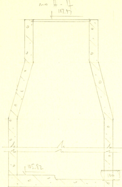
Чертеж колодца М 1:25
