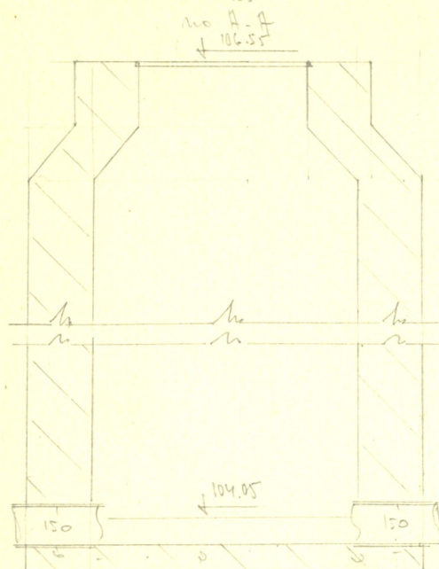
Чертеж колодца М 1:25
