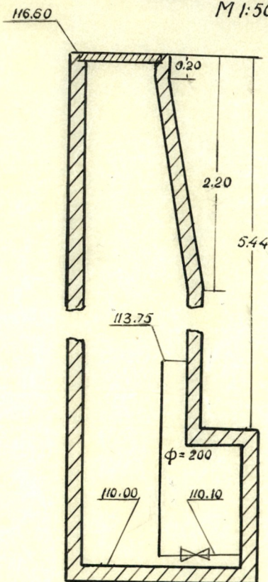
Чертеж колодца М 1:50
