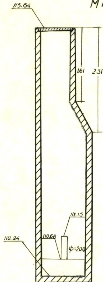
Чертеж колодца М 1:50
