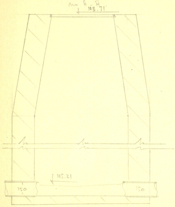
Чертеж колодца М 1: 25
