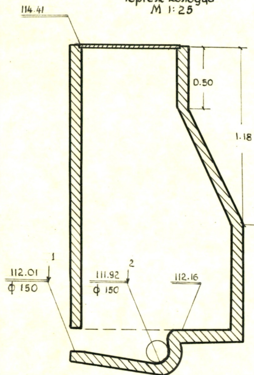
Чертеж колодца М 1:25
