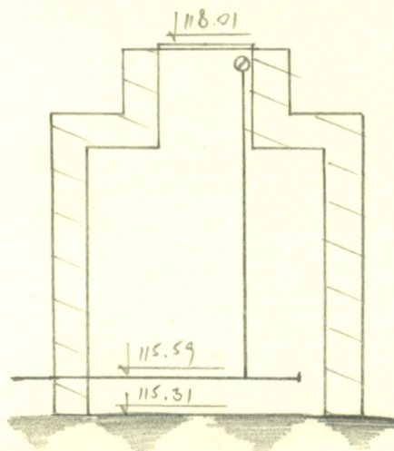
Чертеж колодца М. 1:50
