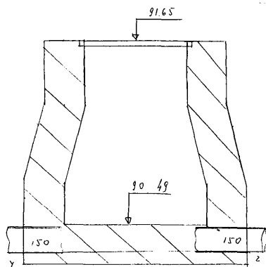
Чертеж колодца М 1:25 по А-А
