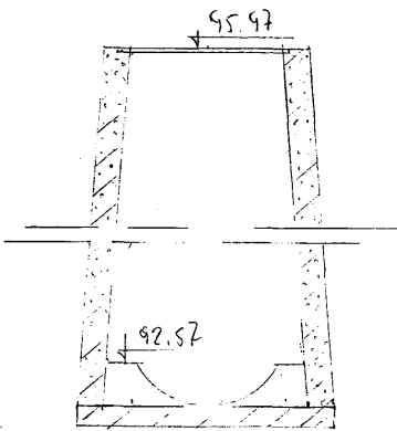
Чертеж колодца М 1:50 По А-А
